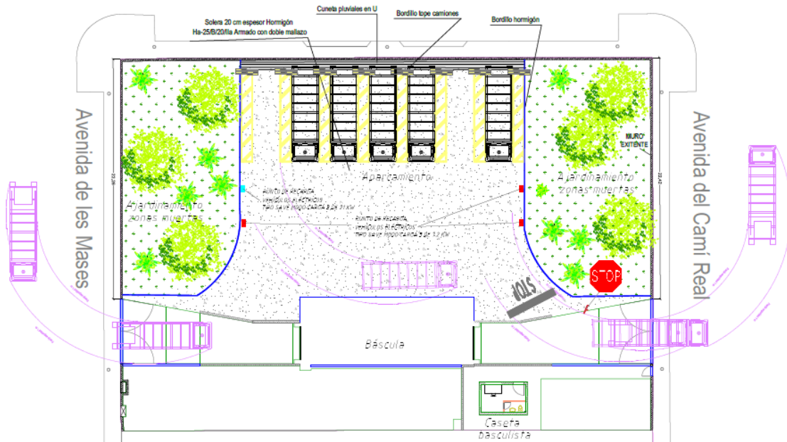
Esquema de base logística de camiones y ecomóviles de Ròtova previsto el Proyecto de Gestión
